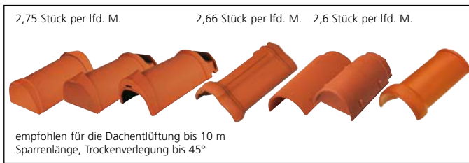
Firstziegel Nr. 19 Firstziegel Nr. 18 Firstziegel Nr. 15 Firstziegel Nr. 21 Standard Walmglocken
